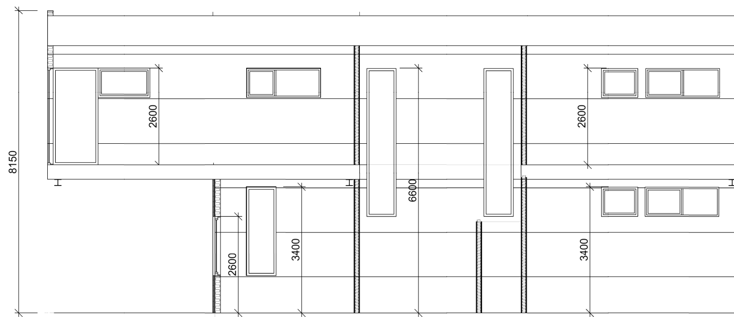
Snitt A_A
